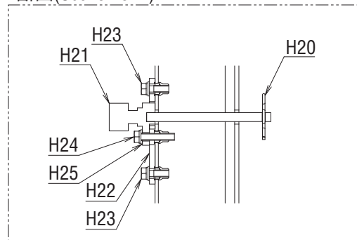
L断面 (Section of L)
